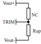
电压上调: 在Trim和输出负之间增加电阻Rup R_{up} = 4.87 / \Delta U - 5.1 ( K \Omega )
