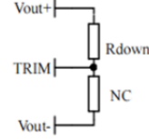
电压下调: 在Trim和输出正之间增加电阻Rdown R_{down} = 1.3 * ( 3.75 - \Delta U ) / \Delta U - 5.1 ( K \Omega )
